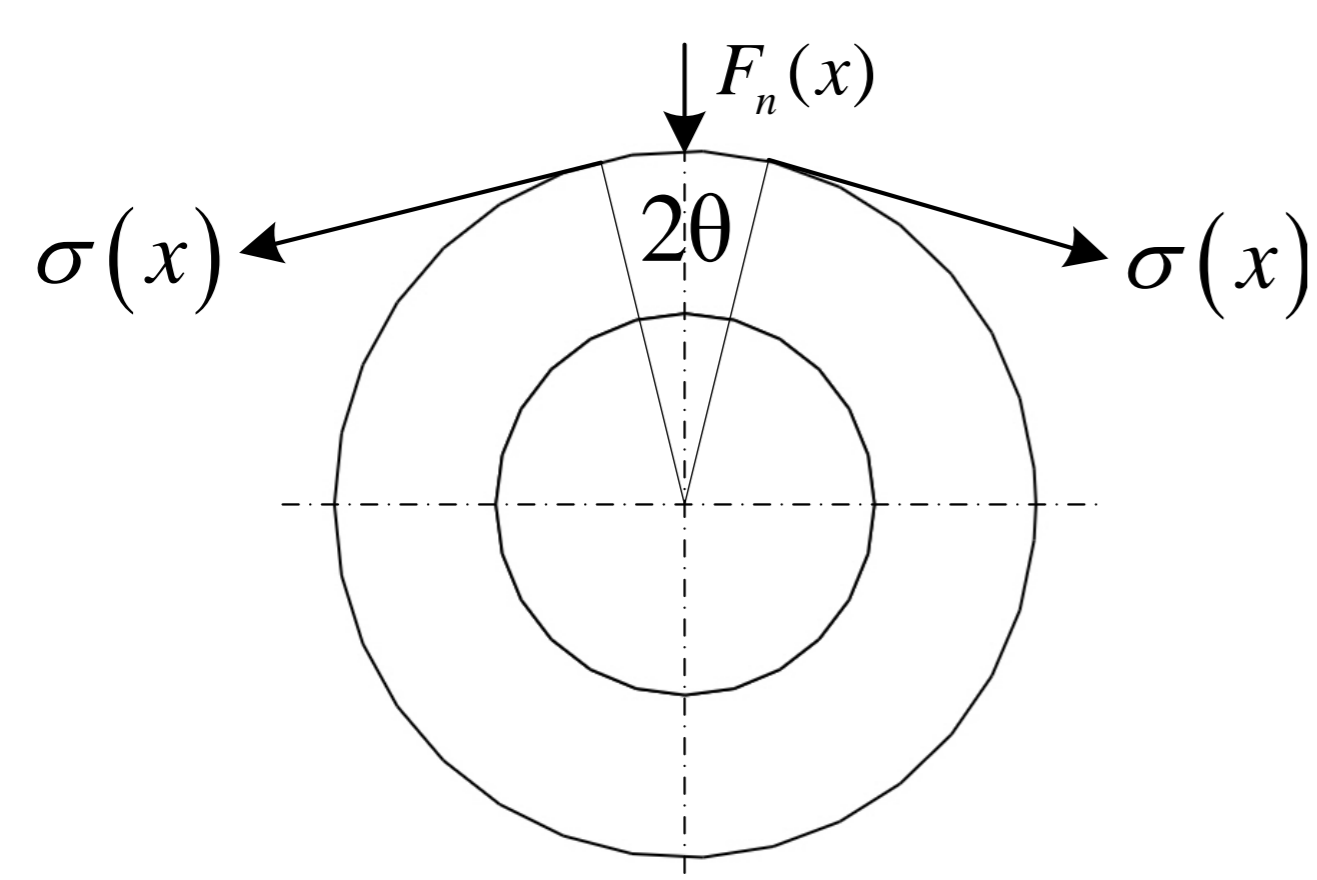
图1 板形检测原理图
