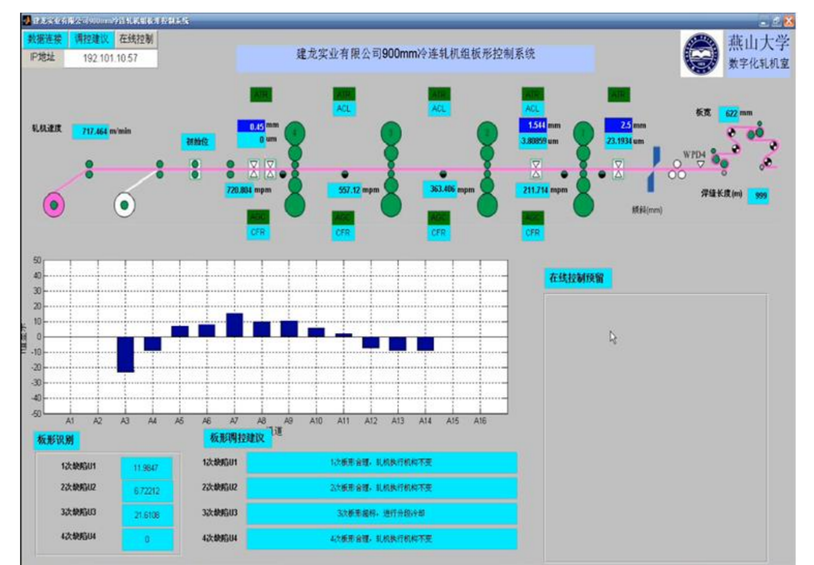
图5 板形控制程序界面
