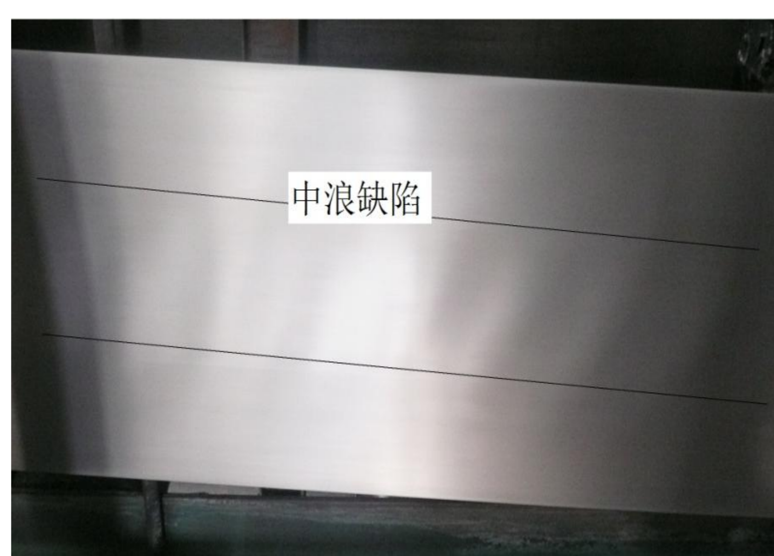
图4 现场脱脂开卷实测中浪缺陷
